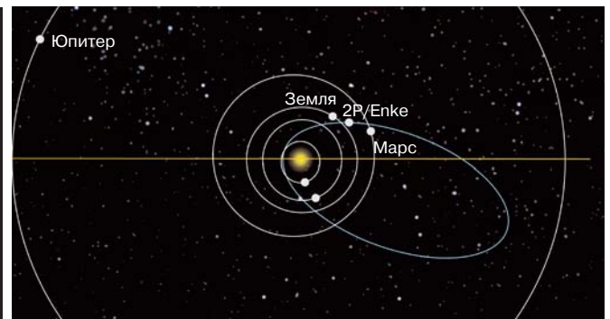
Орбита кометы 2P Энке в солнечной системе и ее положение 17 ноября 2003 года в момент наибольшего сближения с Землей
