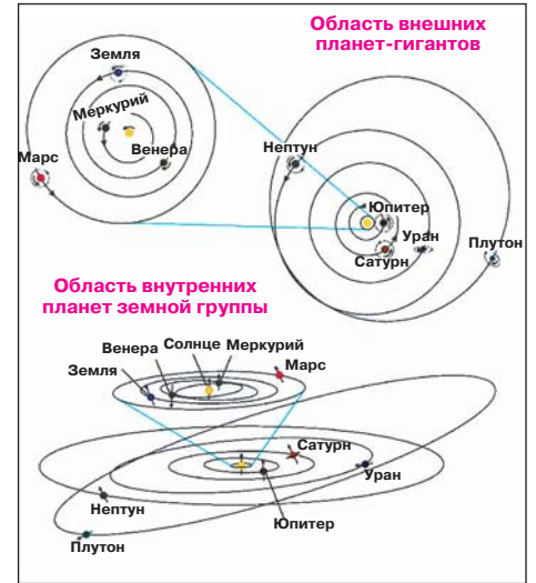
Строение солнечной системы. Сильная вытянутость и большой наклон орбиты Плутона к плоскости эклиптики, а также его малая масса и особенности строения не позволяют отнести его ни к группе планет земного типа, ни к планетам-гигантам.
